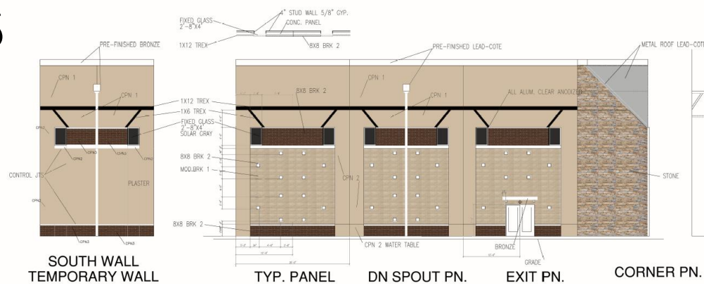
TYP. PANEL
