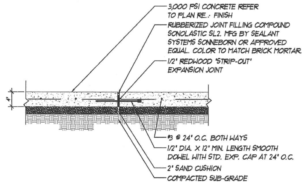
(D) EXPANSION JOINT NOT TO SCALE
