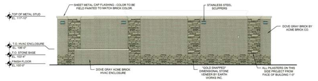
3 WEST ELEVATION A3 SCALE: 1/8" = 1'-0"
