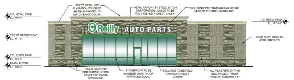
1 EAST ELEVATION A3 SCALE: 1/8" = 1'-0"
