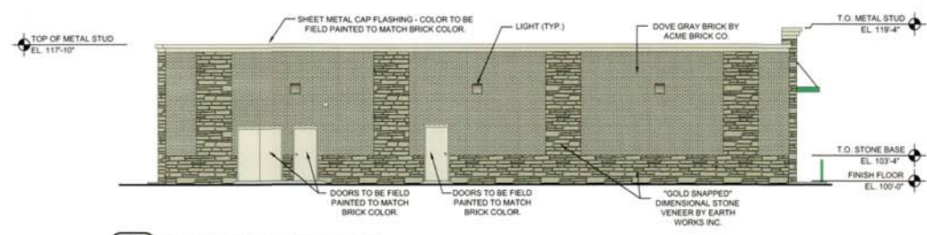
4 SOUTH ELEVATION A3 SCALE: 1/8" = 1'-0"
