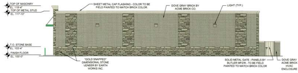
2 NORTH ELEVATION A3 SCALE: 1/8" = 1'-0"
