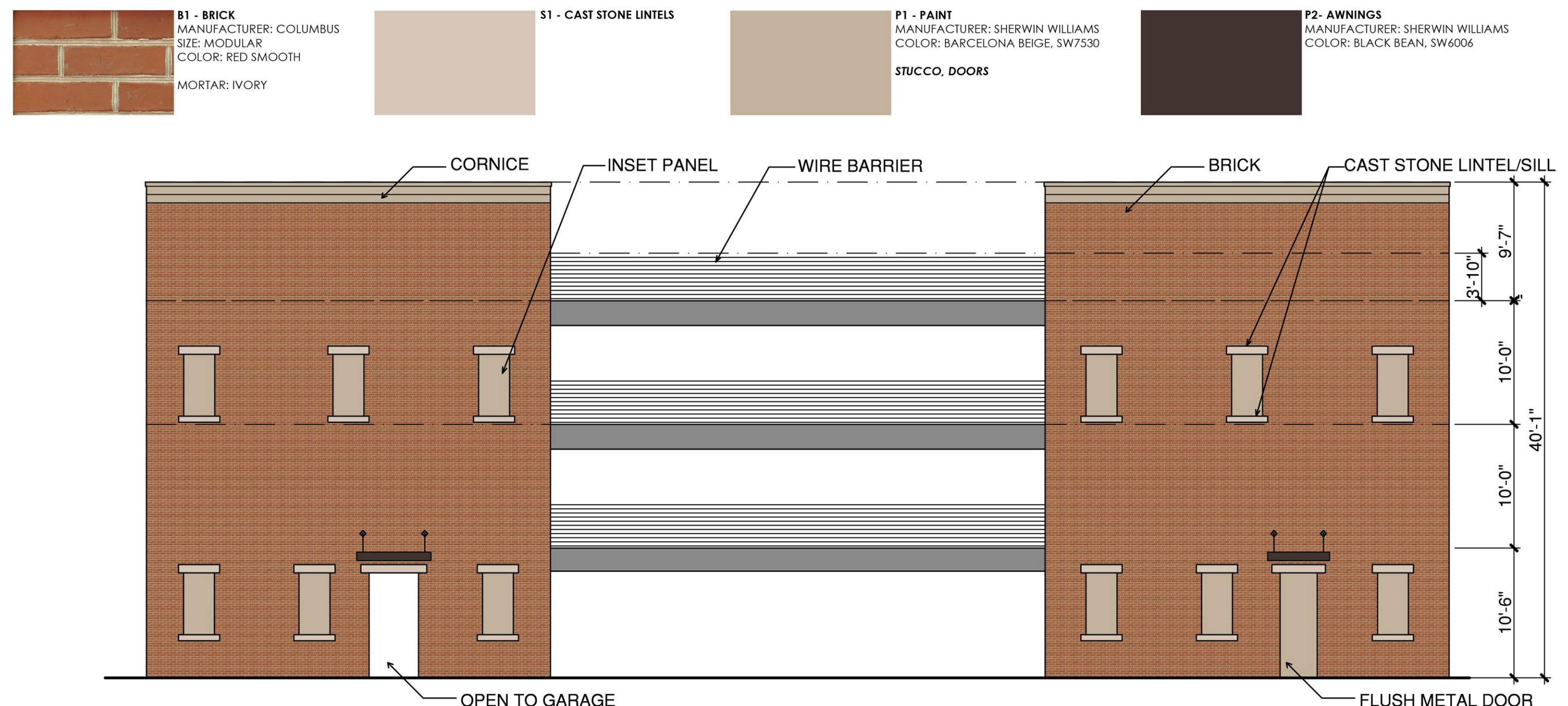
4 WEST GARAGE ELEVATION SCALE: 1/8" = 1'-0"
